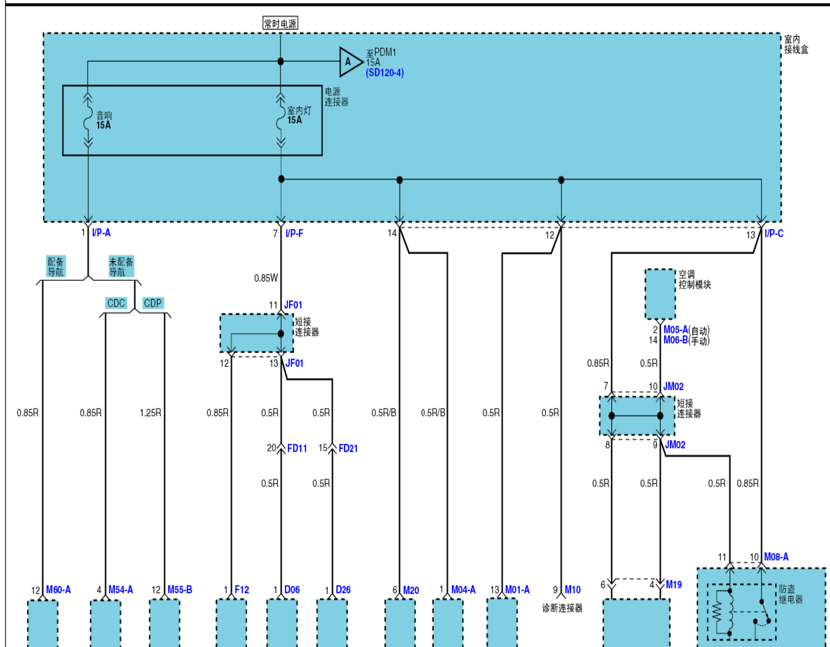
室内保险丝分布(3)
