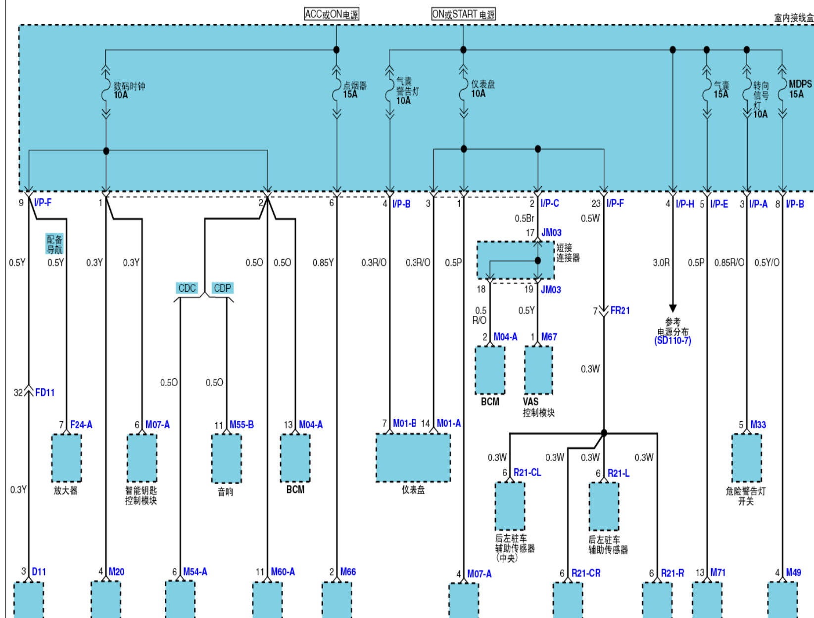
室内保险丝分布(1)
